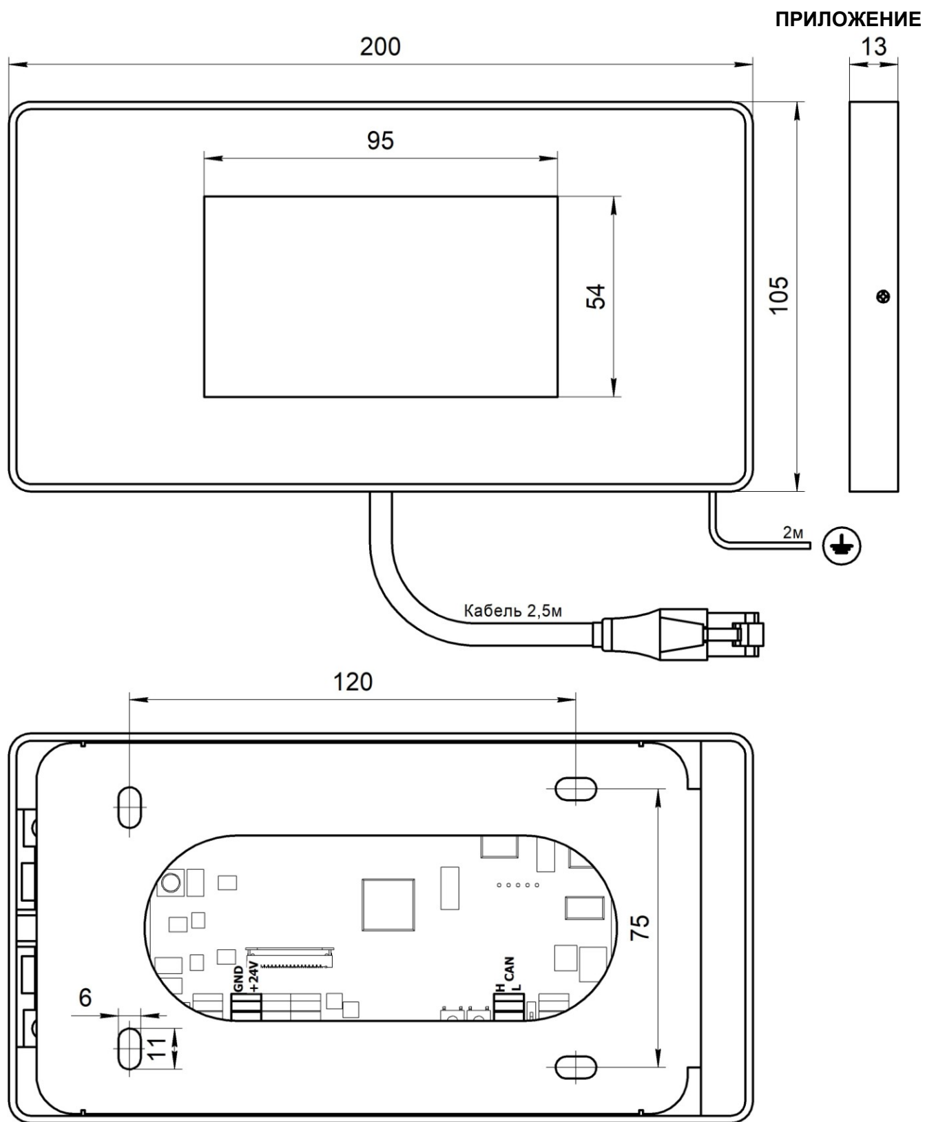
Рис.1 Внешний вид Табло накладное МАЛАХИТ (жгут RJ45) НШЕК.468232.127 (дисплей 4,3)
